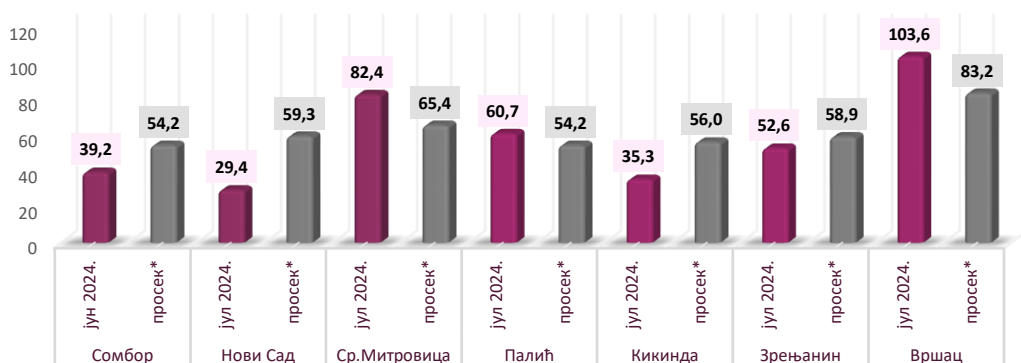
Количина падавина у јулу (у mm) по падавинским станицама у Војводини
